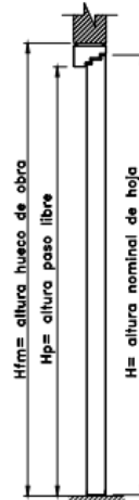
DETALLE A
