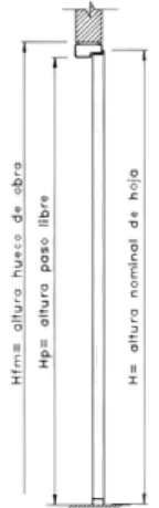
DETALLE A
