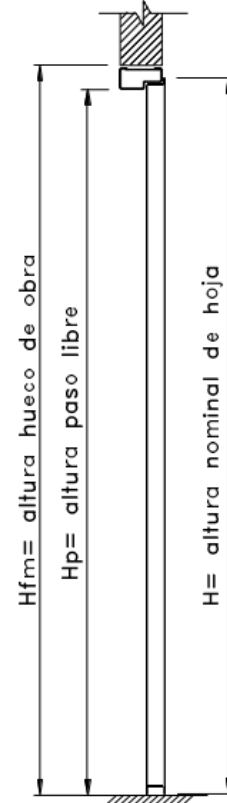
DETALLE A
