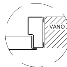
DETALLE A
